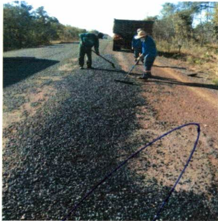
Imagem – Intervenção de tapa buraco em execução TO-446 Abreulândia / Dois Irmãos
